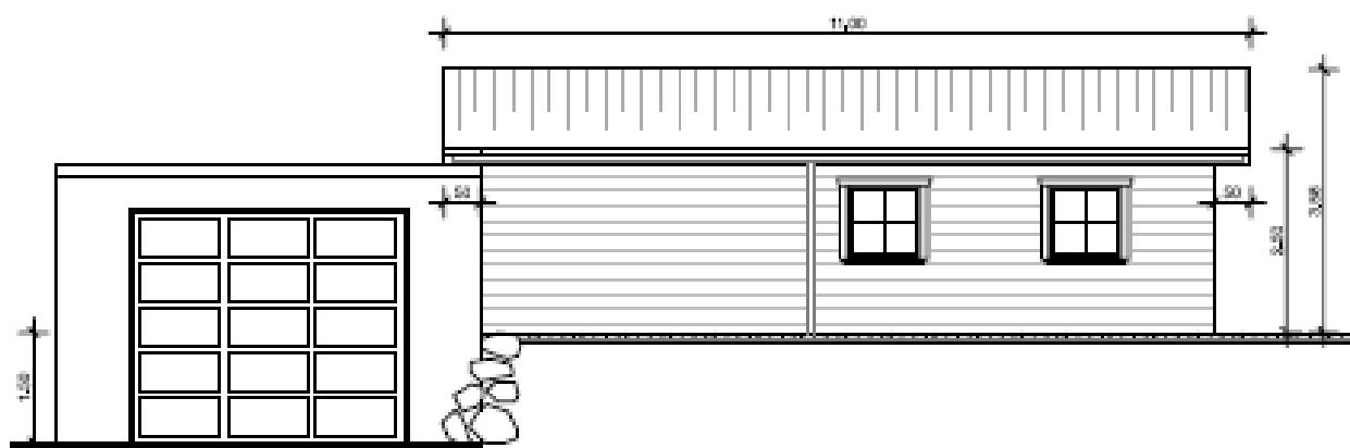
Fassade Nord
